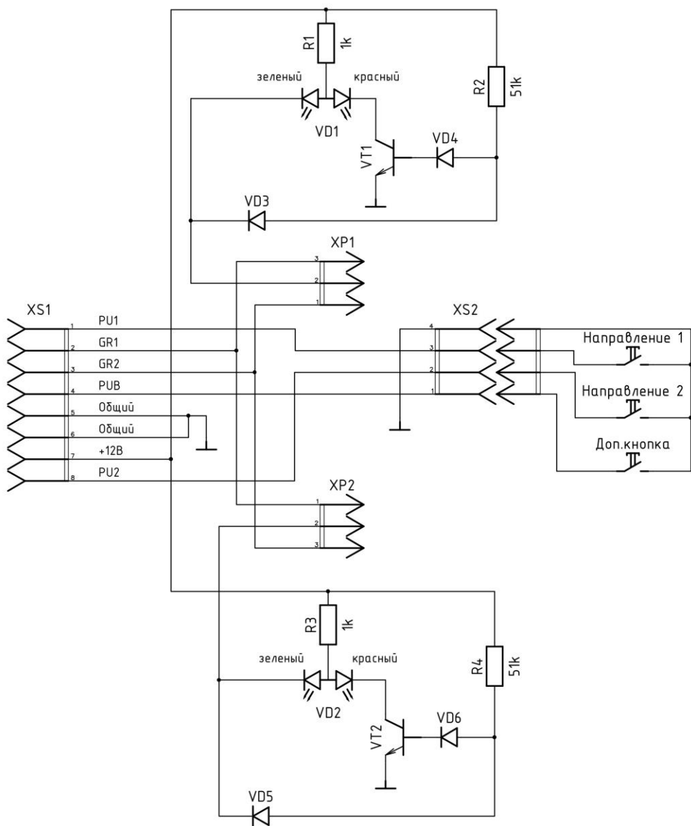
Схема электрическая принципиальная пульт дистанционного П2П-0-0Г
