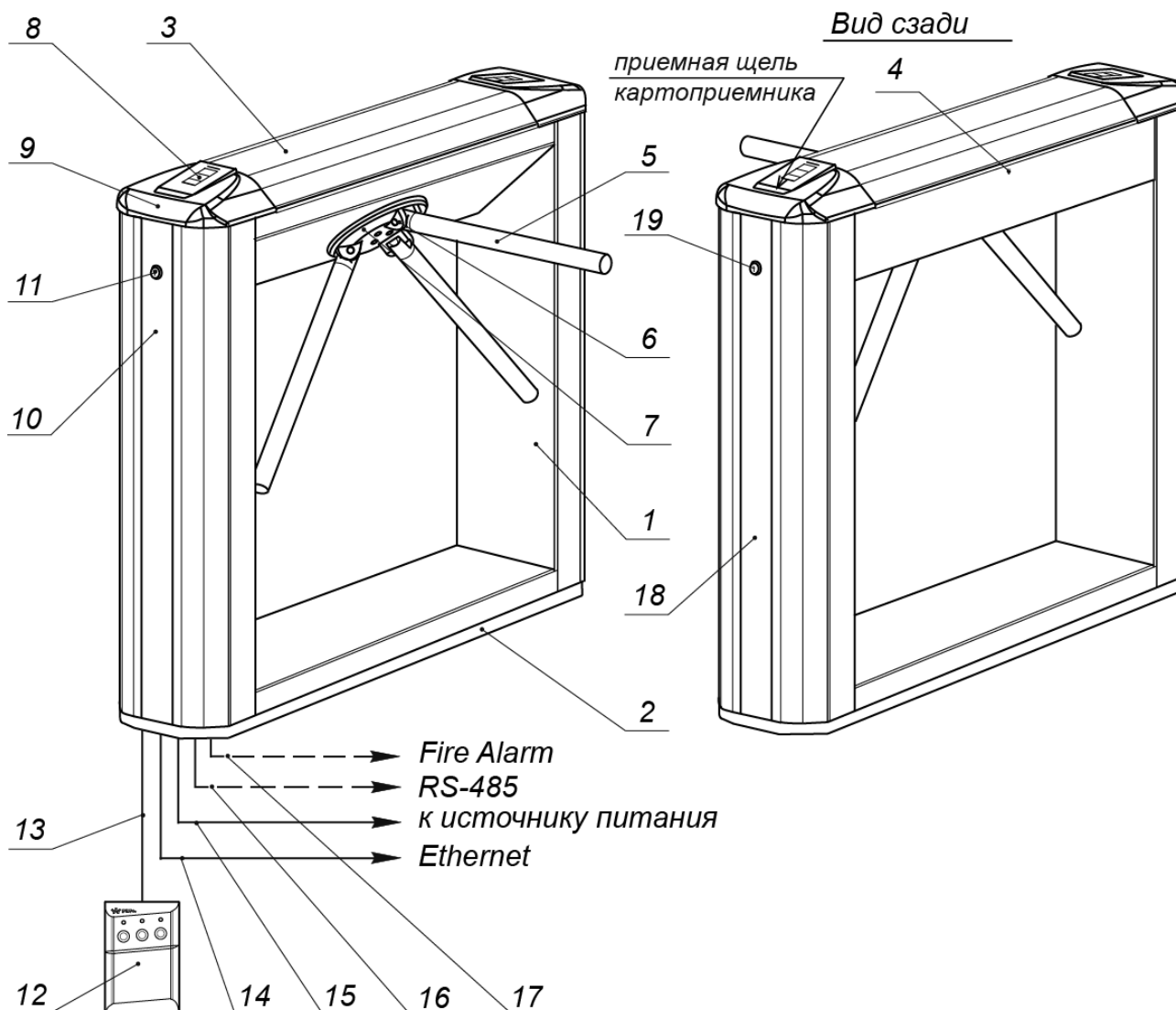
Рисунок 2. Устройство ЭП
