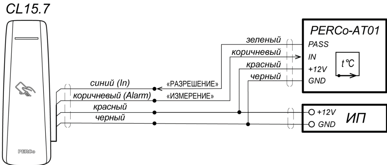
Рисунок 12. Схема подключения пирометра PERCo-AT01 к контроллеру CL15.7
