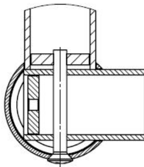
Ограждение угловое L-образное
